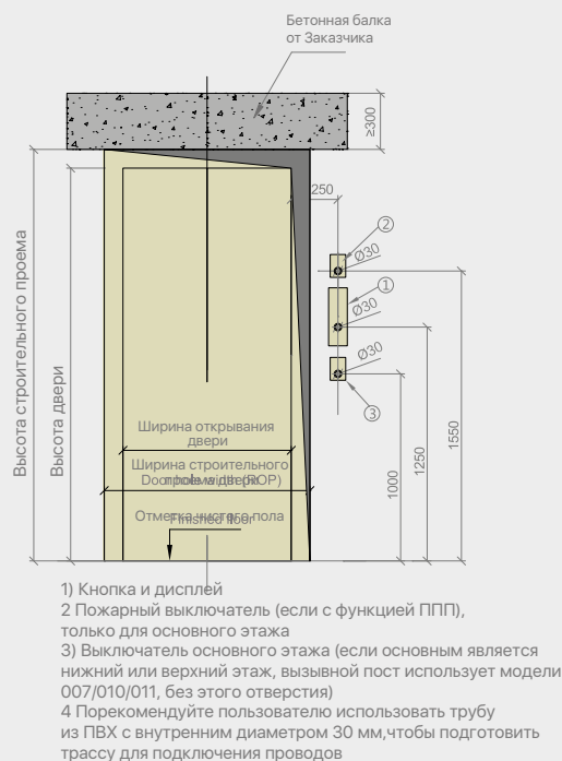
Двери шахты (все этажи)
