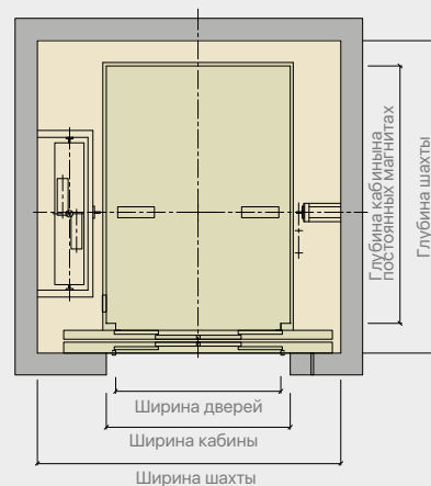
План шахты
