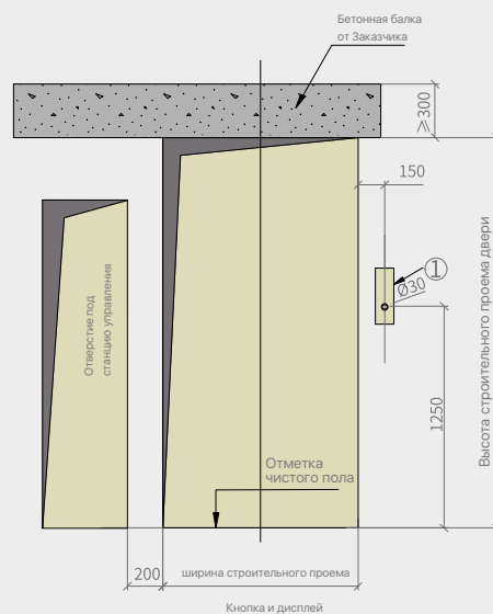
Дверь шахты (верхний этаж)
