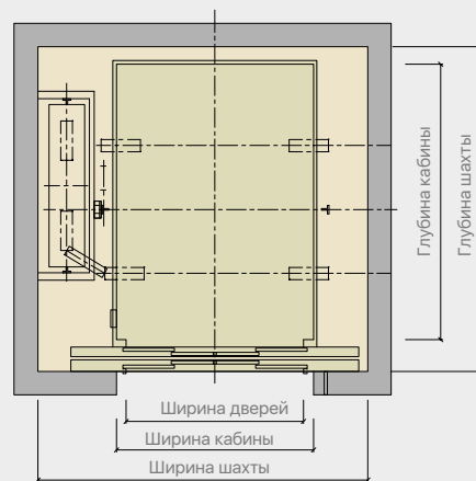
План шахты
