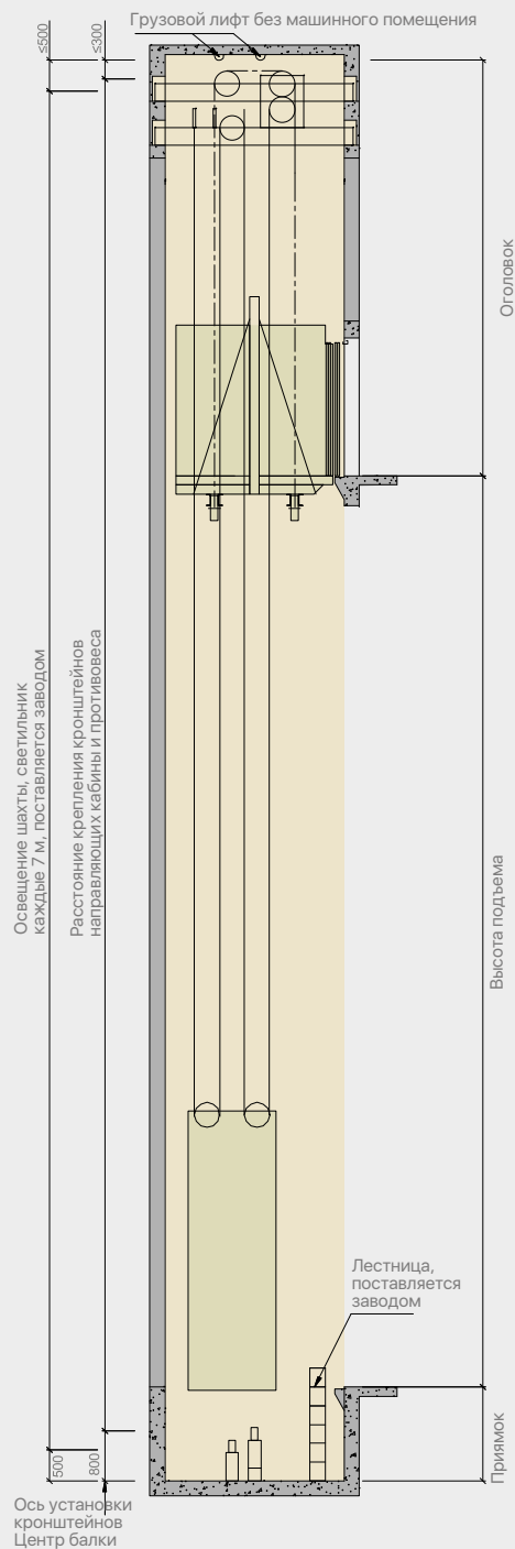
Вертикальный разрез
