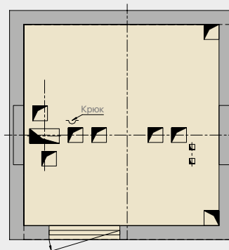
Машинное помещение с подготовленными отверстиями
